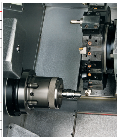
Conjunto porta pinça de troca rápida
